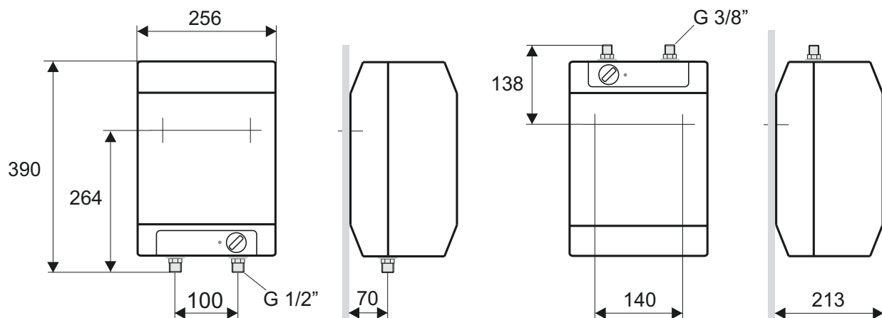
Abb. 1: Über- und Untertischmontage ACK 5 (Maße in mm)
