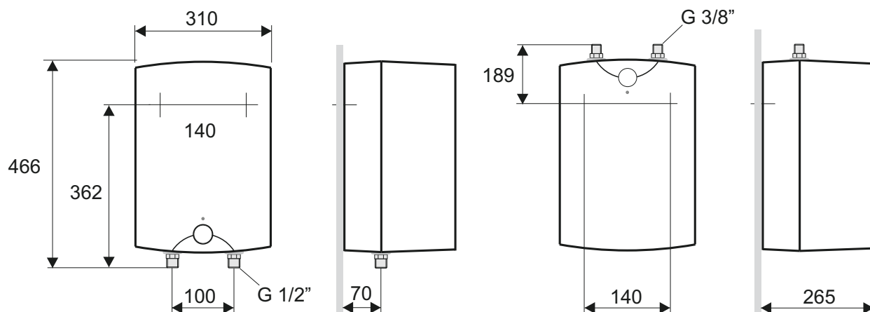
Abb. 2: Über- und Untertischmontage ACK 10 (Maße in mm)
